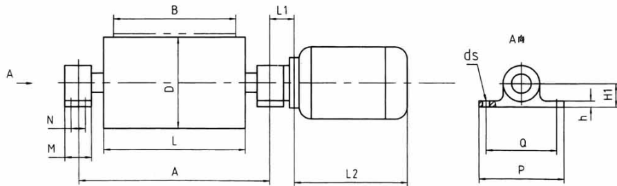
图2 WD II型外装式滚筒
