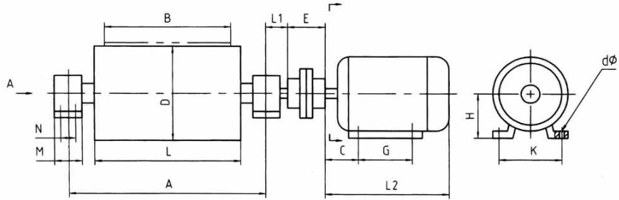
图1 WD I型外装式滚筒
